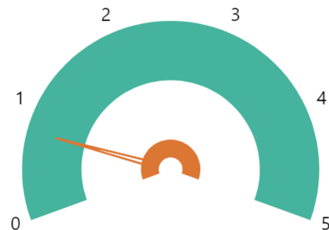
Ranking (quintil)
